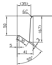
防草溝詳細図
