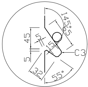
防草目地部詳細図
