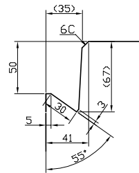
防草溝詳細図
